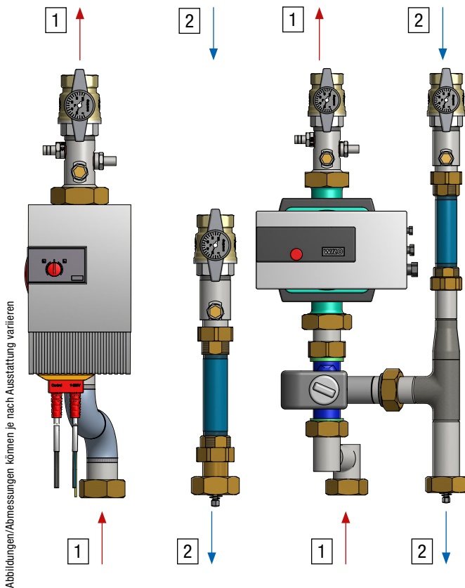
Abbildung pewoHKM SX-Q25: Heizkreismodul, ungemischt (li.), gemischt (re.) Umwälzpumpe ist wählbar, Auswahl siehe Rückseite
